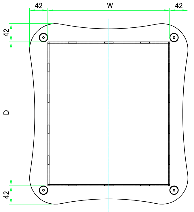
Wパネル1 / W panel 1
